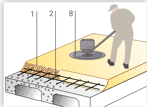
Soletta strutturale con finitura tipo pavimento industriale
