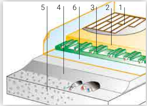
Massetto radiante su pannelli tradizionali ( \geq 1 cm sopra tubo/bugna).
