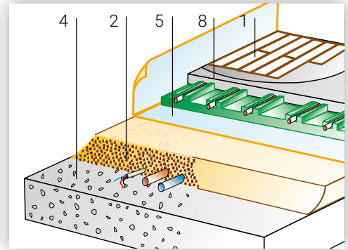
Rasamento impianti per la posa di sistemi di riscaldamento a pavimento.
