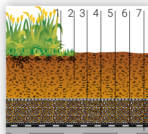
Strati drenanti e permeabili all'acqua.
