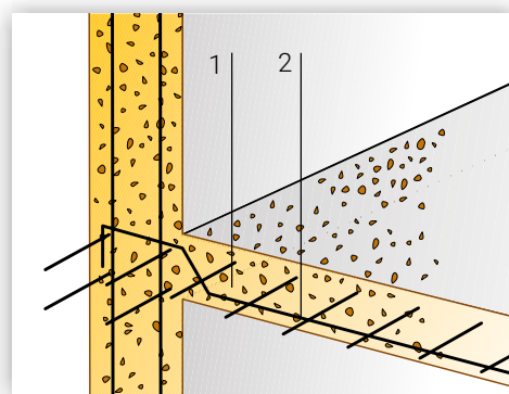
Getti strutturali.
