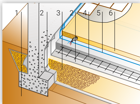
Vespaio contro terra.
