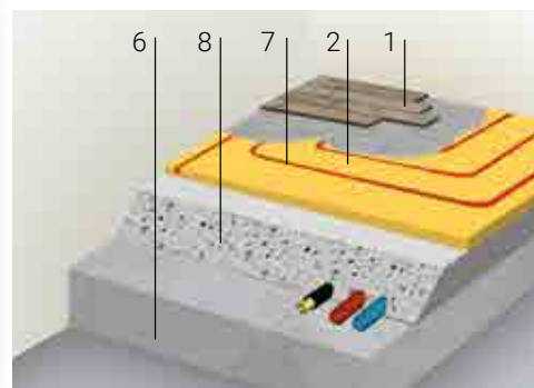
Pavimenti radianti di tipo fresato.
